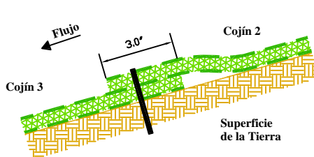
Figura B - Vista de Perfil
